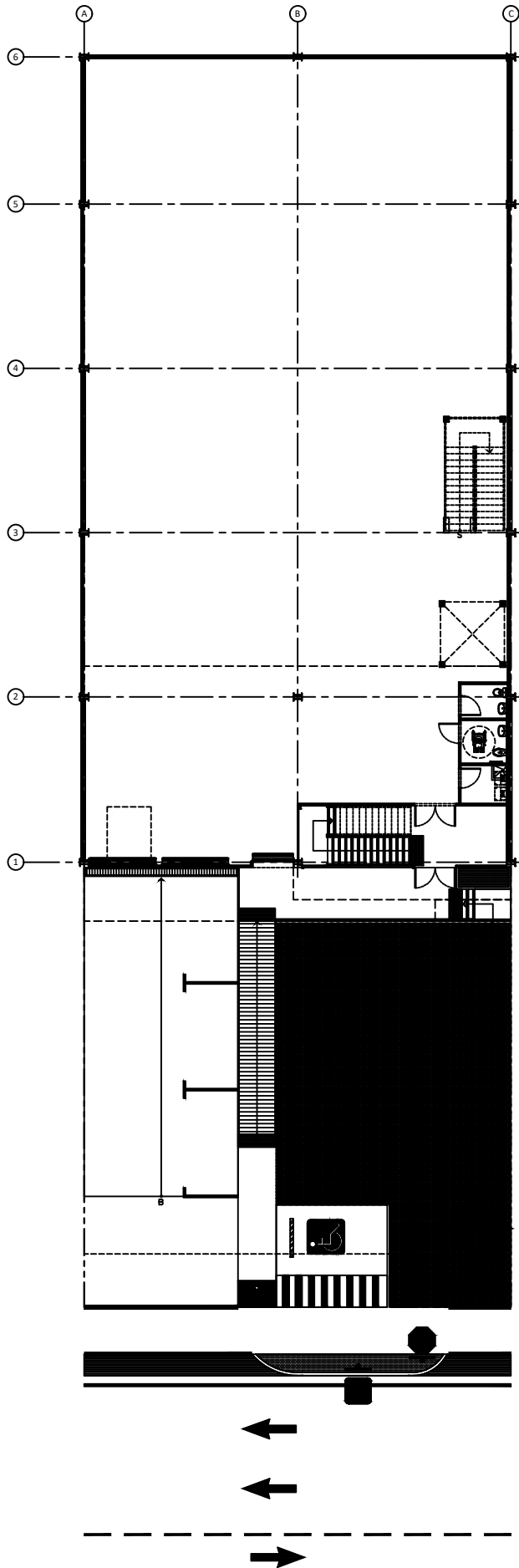
PLANTA ARQUITECTÓNICA PLANTA BAJA - NIV. 000 BODEGA TIPO B ESCALA 1:100
